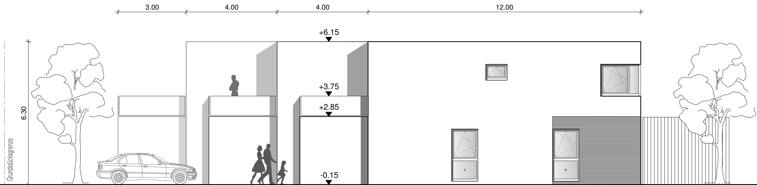
ANSICHT NORD
