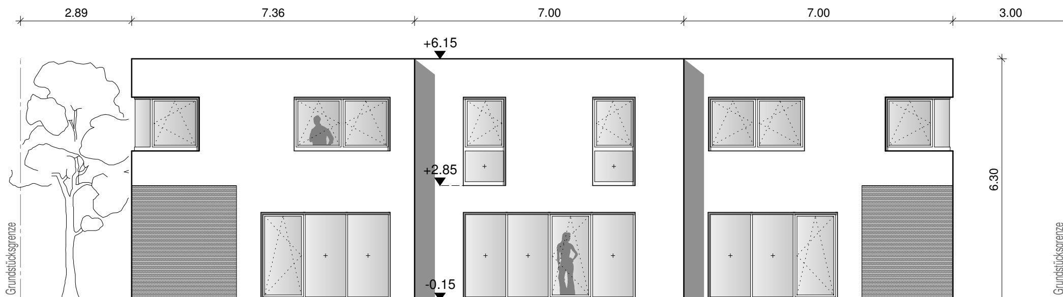
ANSICHT WEST (GARTEN)
